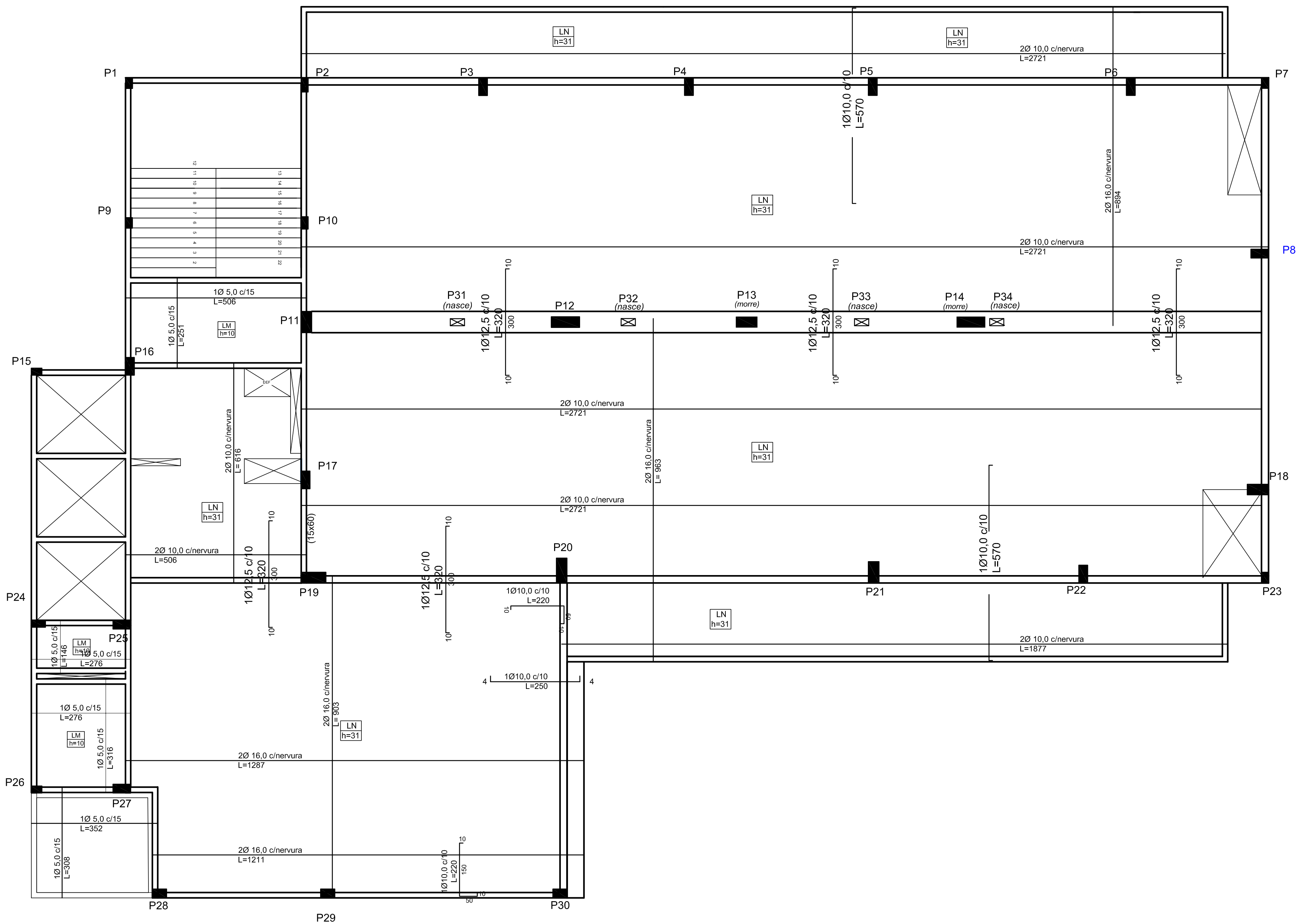
Planta de Fôrmas 4º Pavimento - Ferragem Escala 1:75
